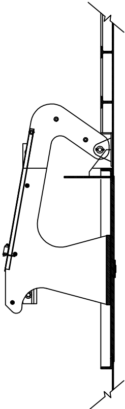
Corte A-A Detalle Escotilla
