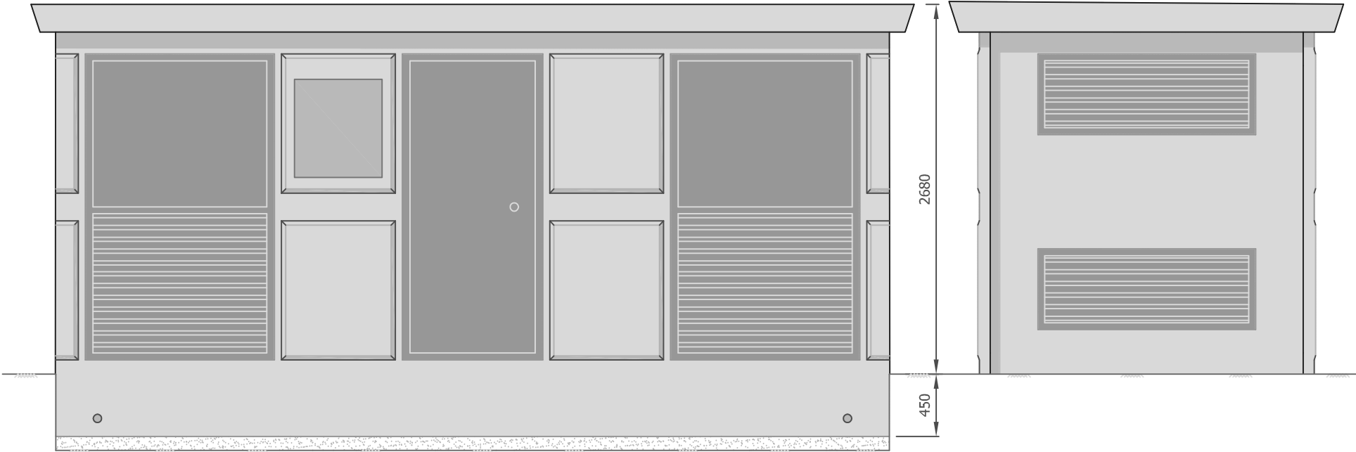
Vista Panel Frontal y Lateral Ventana PAMPA 3 DU/T3
